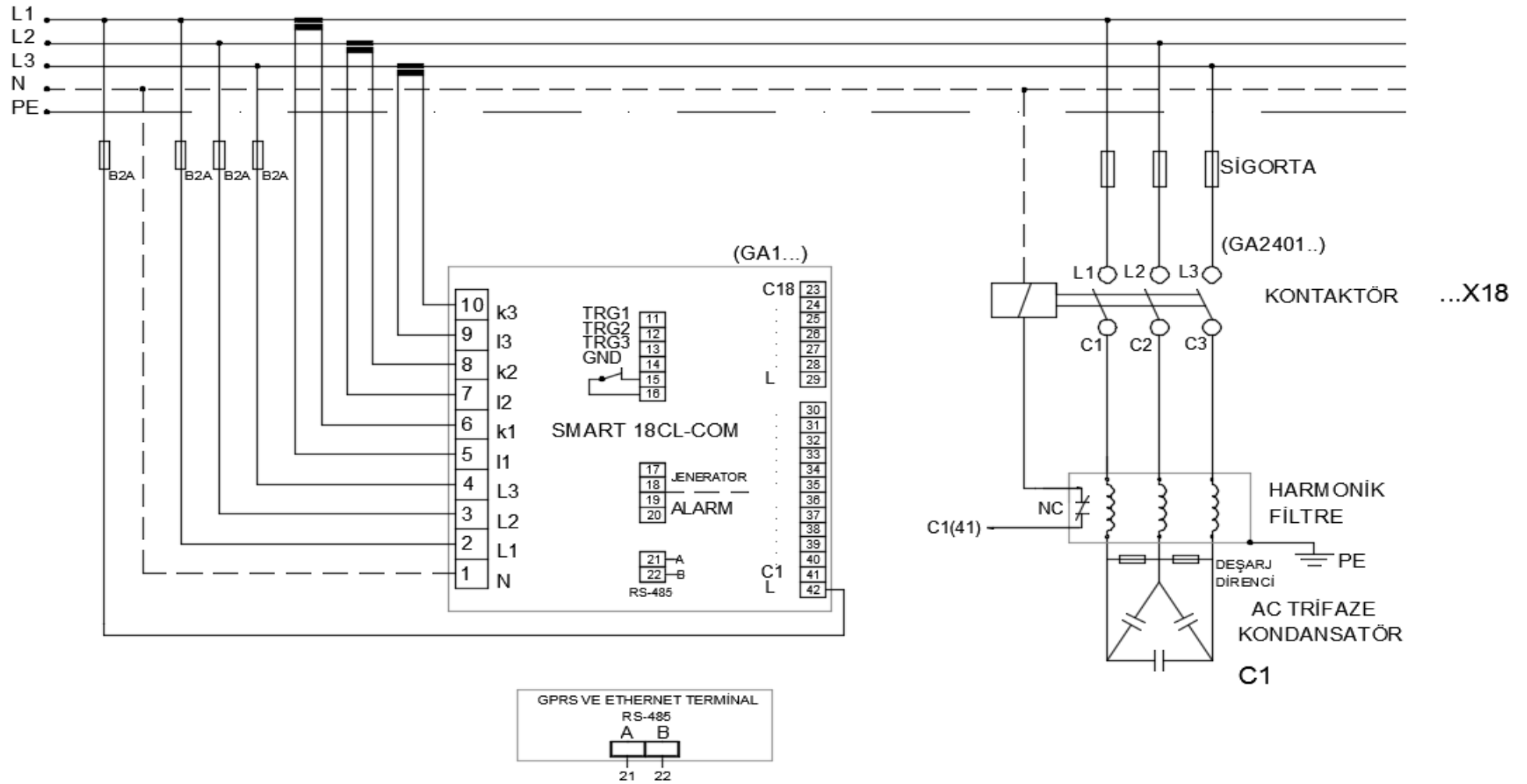
Smart 18 CL-COM Bağlantı Şeması
