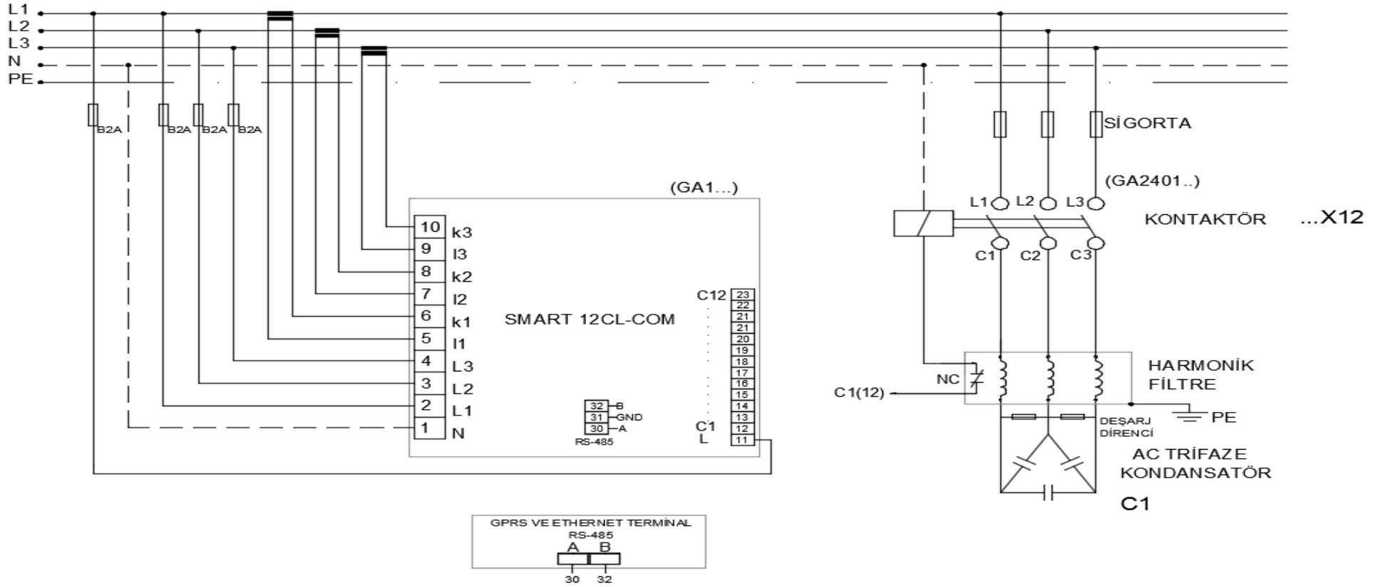
Smart 12 CL-COM Bağlantı Şeması
